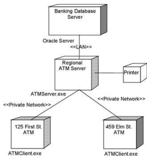
Рис. 19. Пример диаграммы размещения
