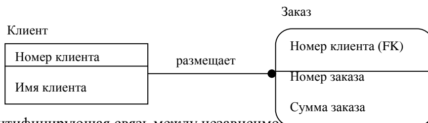
Рис. 5. Идентифицирующая связь между независимой и зависимой сущностью.
