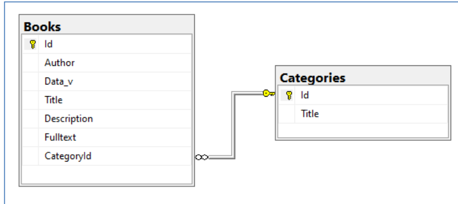
Рисунок 1. ERD-диаграмма
